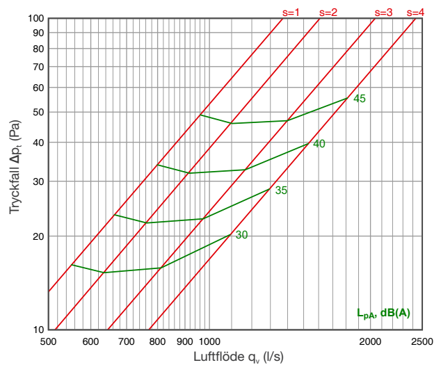
Frånluft: HU L=5500...5900
