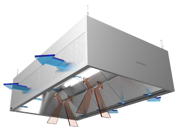
Ångfälla, med tilluft
