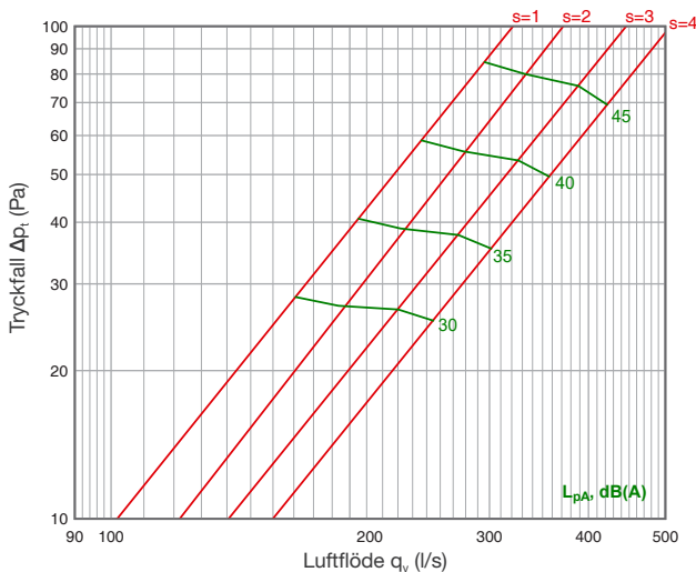
Frånluft: HU L=1000...1400
