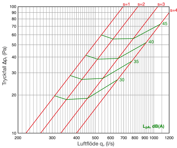
Frånluft: HU L=3000...3400
