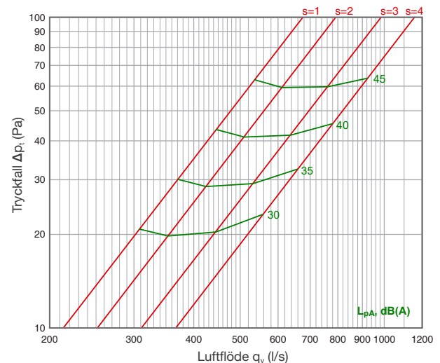
Frånluft: HU L=2500...2900
