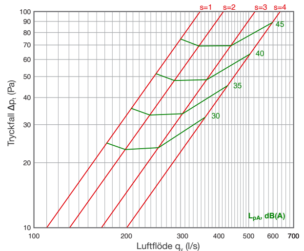
Frånluft: HU L=1500...1900
