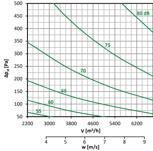
Diagramm nr. 16 – 500 × 400
