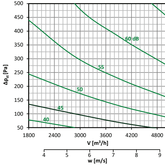
Diagramm nr. 42 – 600 × 250
