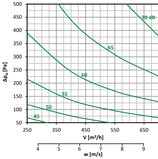
Diagramm nr. 1 – 200 × 100
