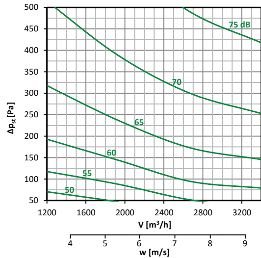
Diagramm nr. 10 – 400 × 250
