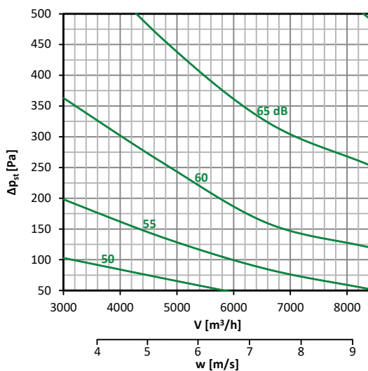
Diagramm nr. 40 – 500 × 400
