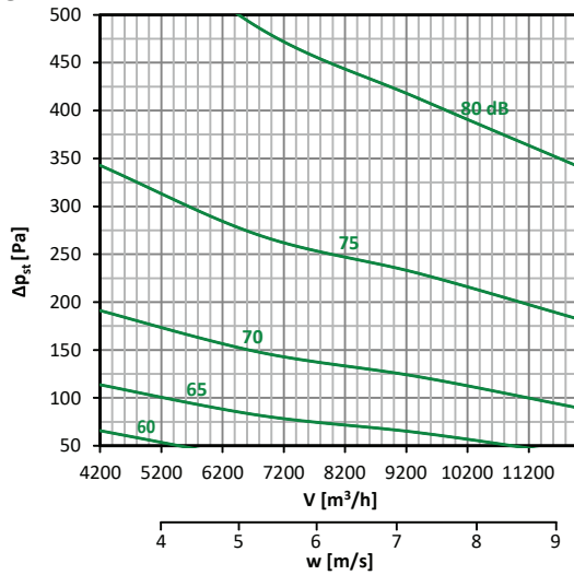
Diagramm nr. 23 – 600 × 600
