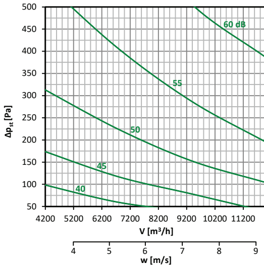
Diagramm nr. 69 – 600 × 600
