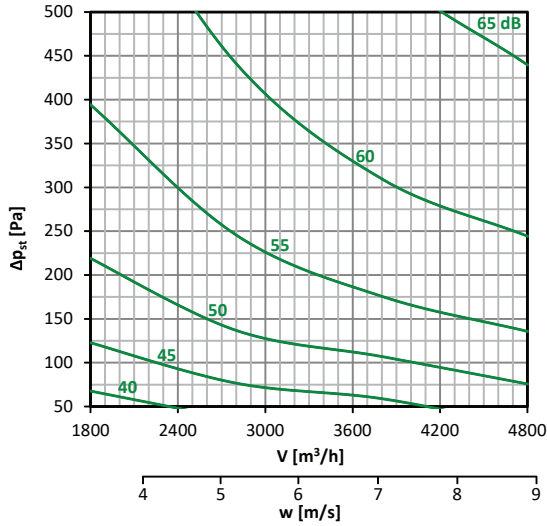
Diagramm nr. 38 – 500 × 300
