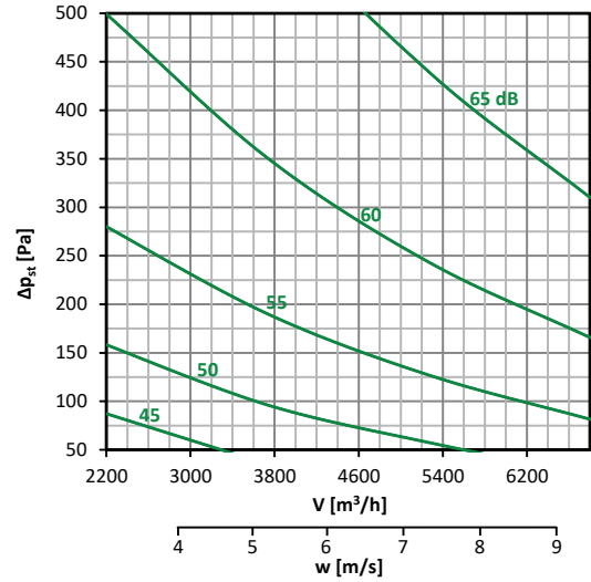
Diagramm nr. 39 – 500 × 400
