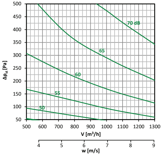
Diagramm nr. 3 – 200 × 100
