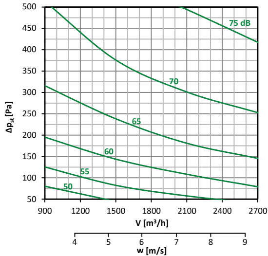
Diagramm nr. 9 – 400 × 200
