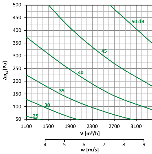
Diagramm nr. 59 – 500 × 200
