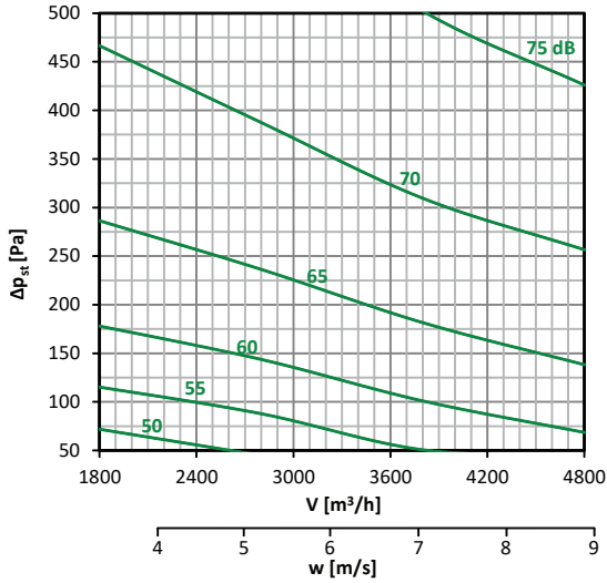
Diagramm nr. 15 – 500 × 300
