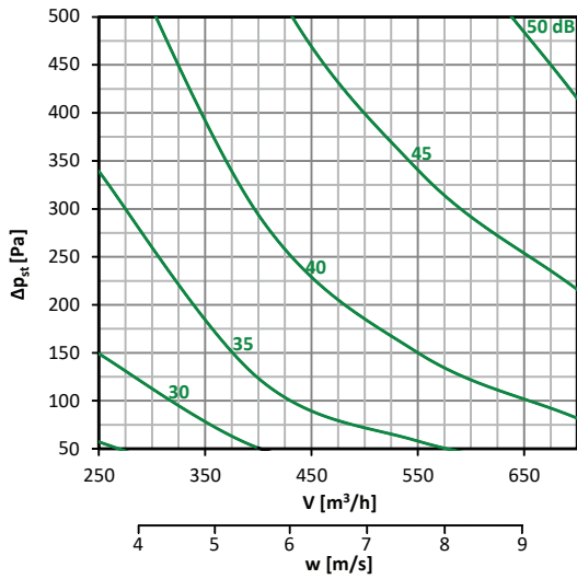
Diagramm nr. 47 – 200 × 100
