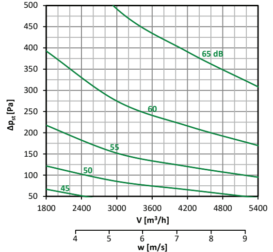
Diagramm nr. 35 – 400 × 400
