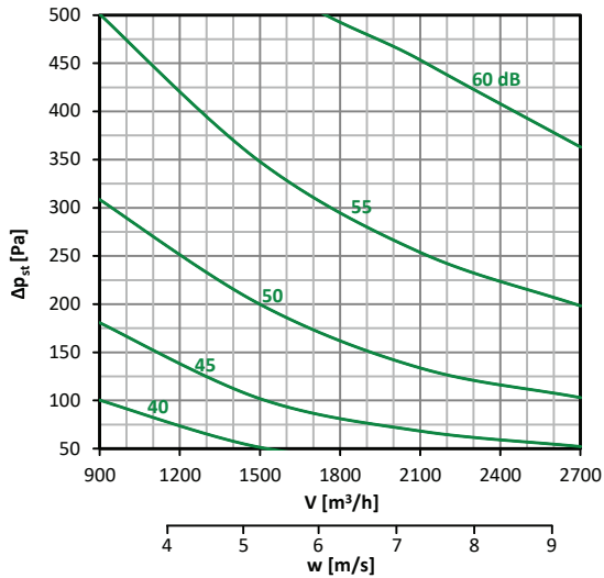
Diagramm nr. 32 – 400 × 200
