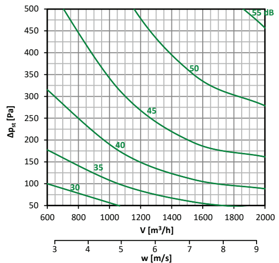
Diagramm nr. 52 – 300 × 200
