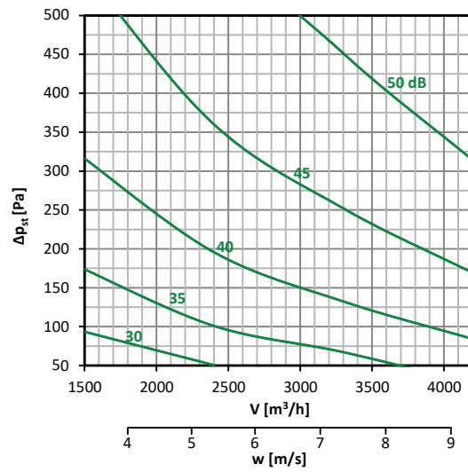
Diagramm nr. 60 – 500 × 250
