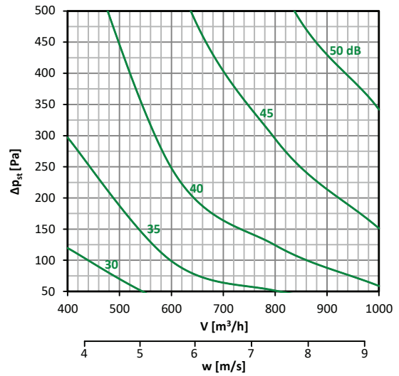
Diagramm nr. 48 – 200 × 150
