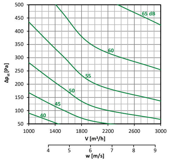
Diagramm nr. 31 – 300 × 300
