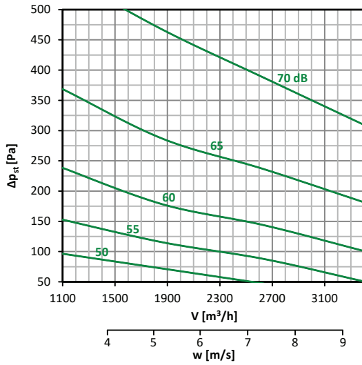
Diagramm nr. 13 – 500 × 200
