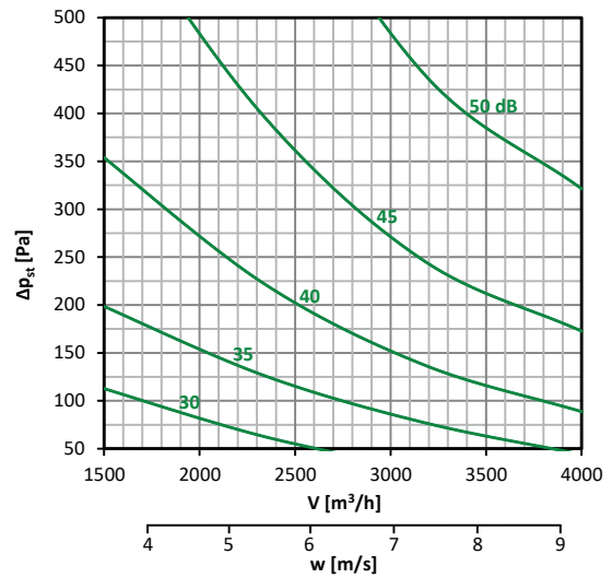
Diagramm nr. 64 – 600 × 200
