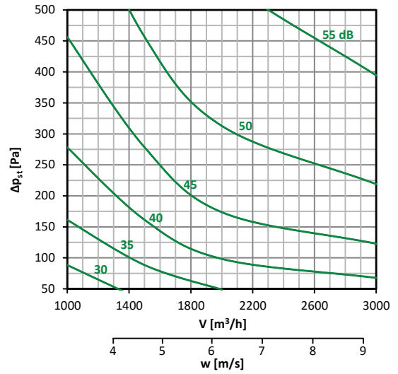
Diagramm nr. 54 – 300 × 300
