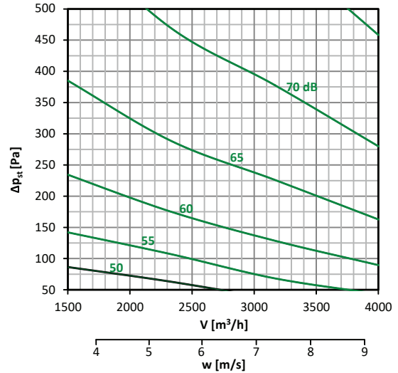
Diagramm nr. 18 – 600 × 200
