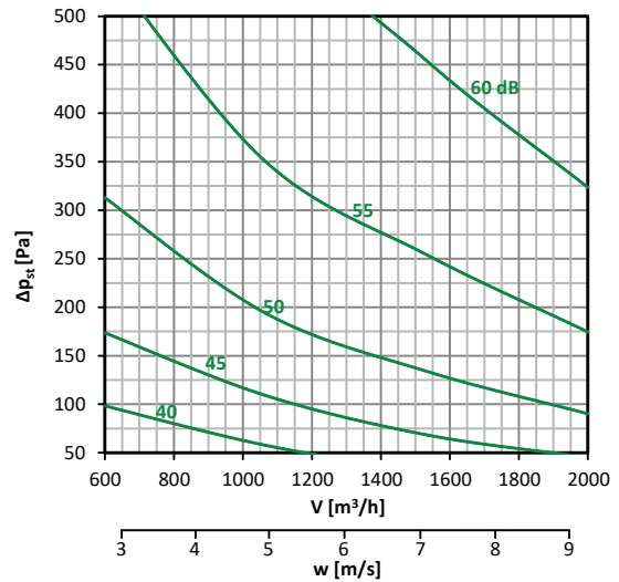
Diagramm nr. 29 – 300 × 200
