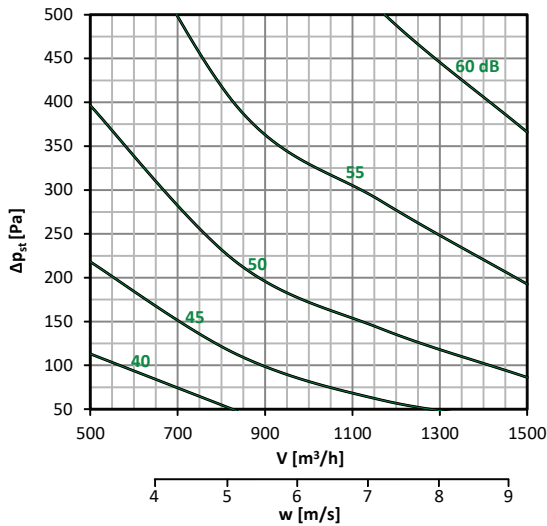
Diagramm nr. 28 – 300 × 150
