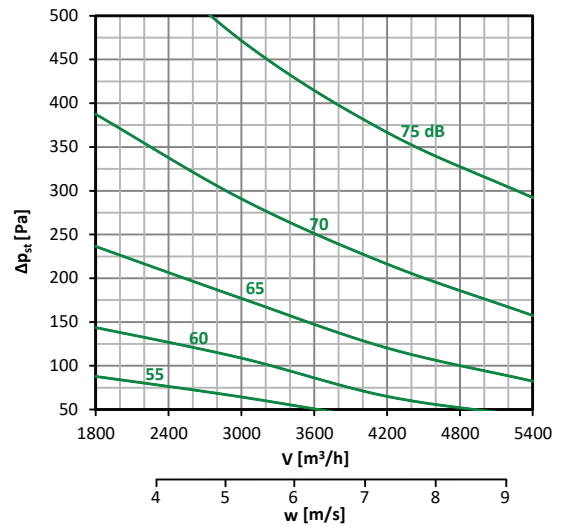
Diagramm nr. 12 – 400 × 400
