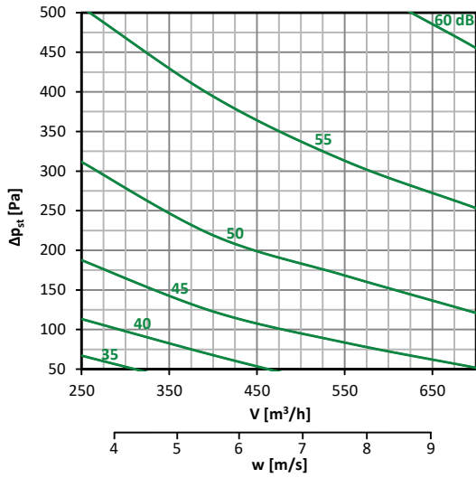
Diagramm nr. 24 – 200 × 100
