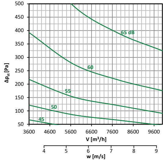
Diagramm nr. 45 – 600 × 500
