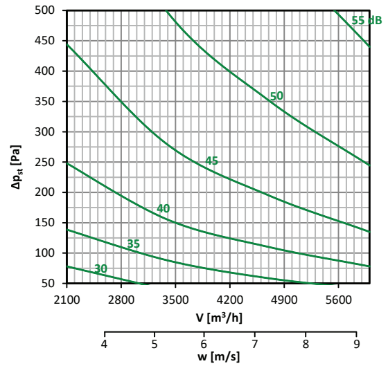
Diagramm nr. 66 – 600 × 300
