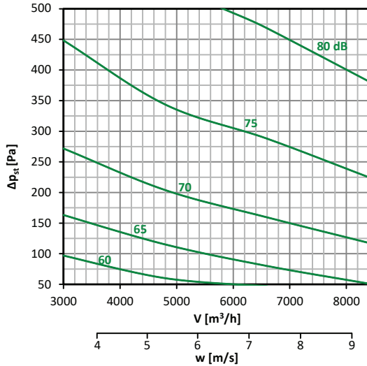
Diagramm nr. 17 – 500 × 500
