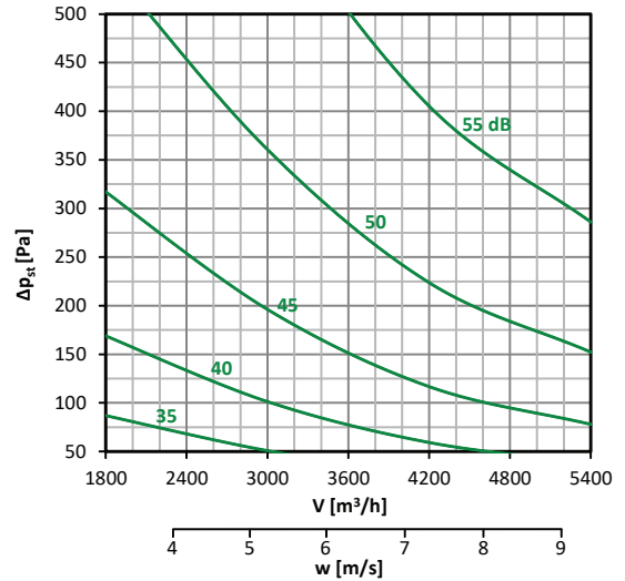
Diagramm nr. 58 – 400 × 400
