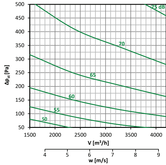
Diagramm nr. 14 – 500 × 250
