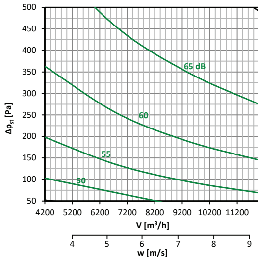
Diagramm nr. 46 – 600 × 600
