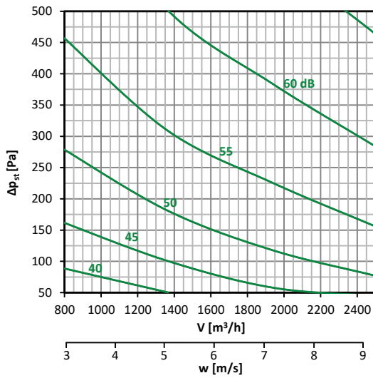
Diagramm nr. 30 – 300 × 250
