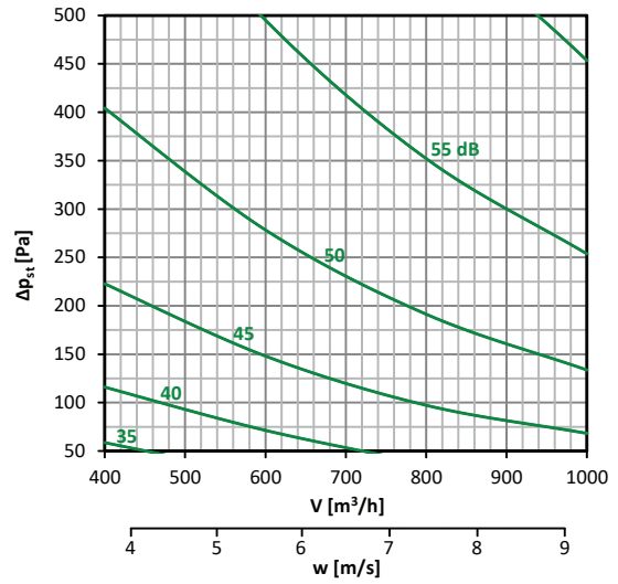
Diagramm nr. 25 – 200 × 150
