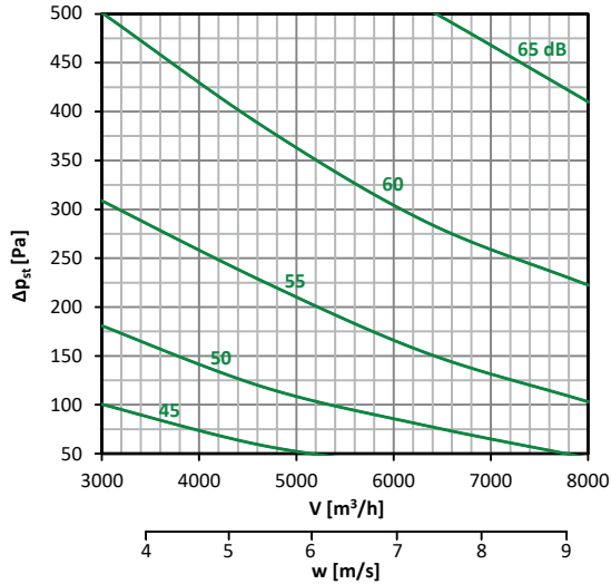
Diagramm nr. 44 – 600 × 400
