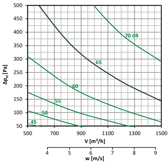
Diagramm nr. 5 – 300 × 150
