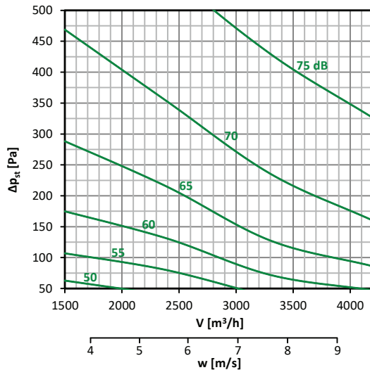
Diagramm nr. 11 – 400 × 300
