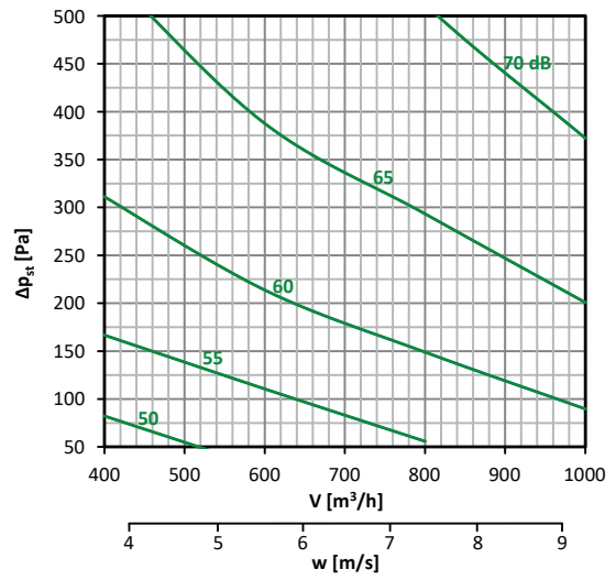
Diagramm nr. 4 – 300 × 100
