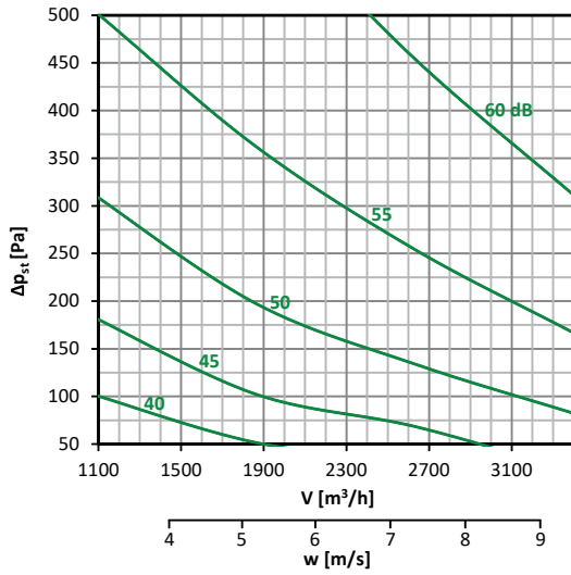
Diagramm nr. 36 – 500 × 200
