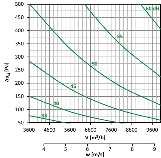
Diagramm nr. 68 – 600 × 500
