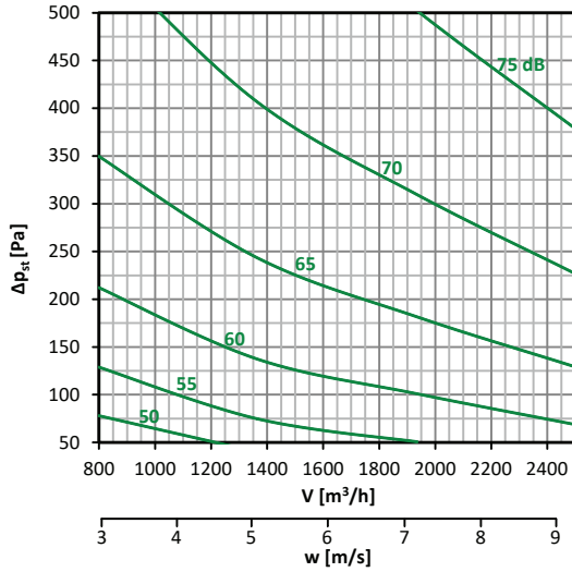
Diagramm nr. 7 – 300 × 250
