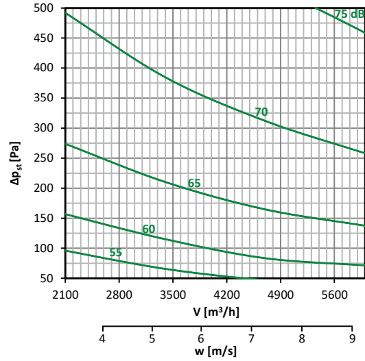
Diagramm nr. 20 – 600 × 300
