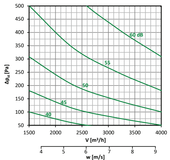
Diagramm nr. 41 – 600 × 200
