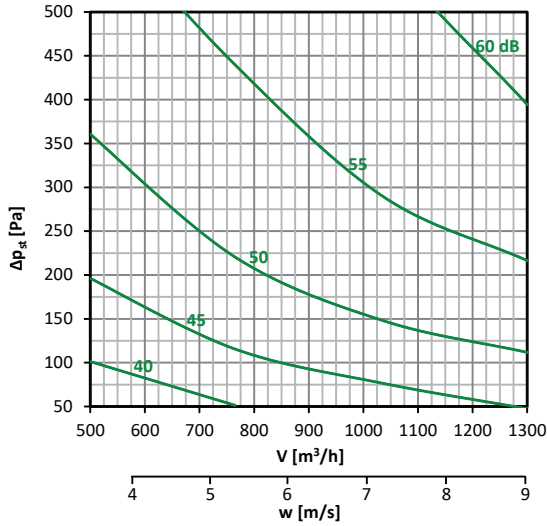
Diagramm nr. 26 – 200 × 200
