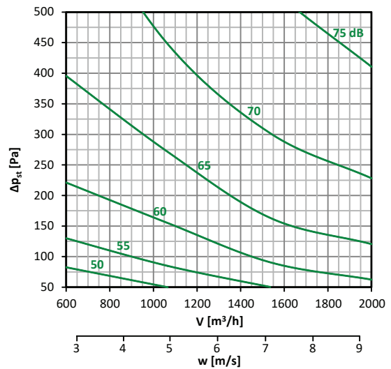
Diagramm nr. 6 – 300 × 200
