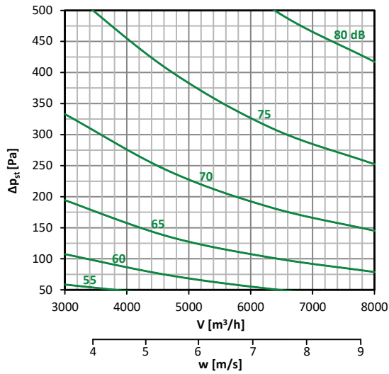
Diagramm nr. 21 – 600 × 400
