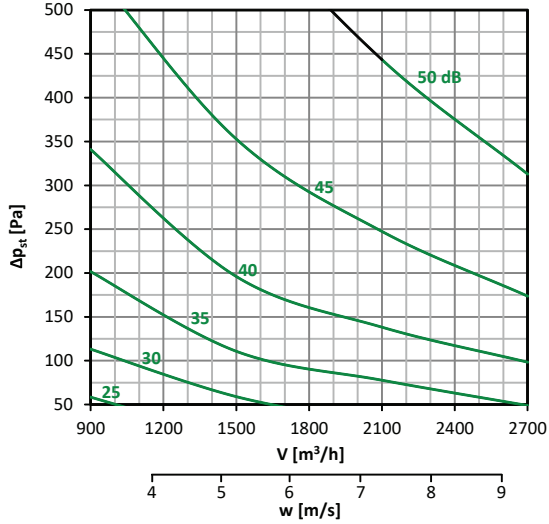
Diagramm nr. 55 – 400 × 200
