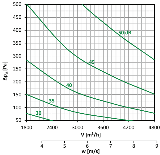
Diagramm nr. 61 – 500 × 300
