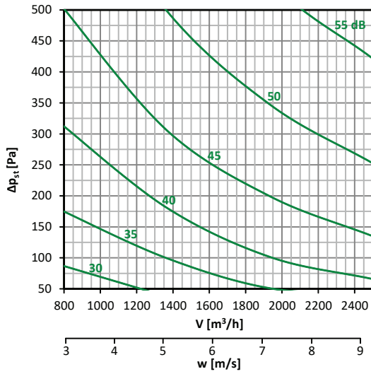
Diagramm nr. 53 – 300 × 250
