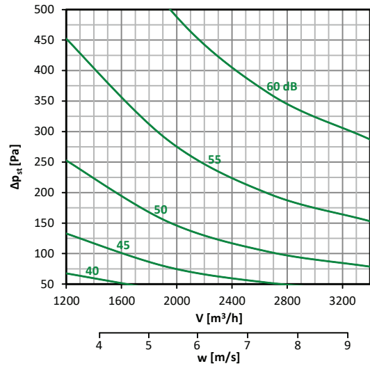
Diagramm nr. 33 – 400 × 250
