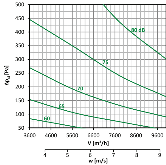
Diagramm nr. 22 – 600 × 500
