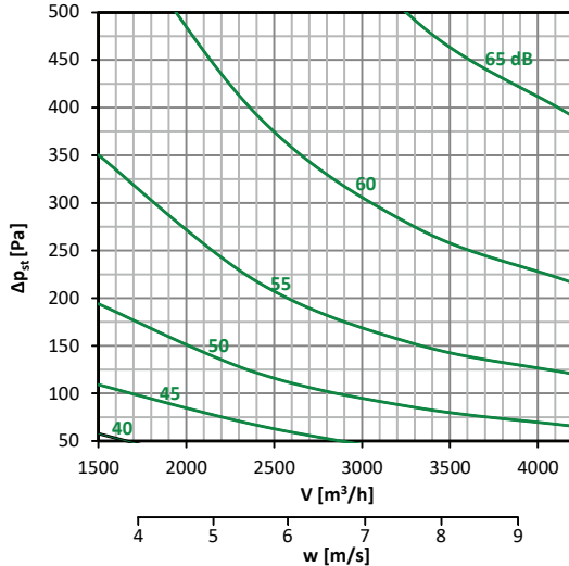
Diagramm nr. 34 – 400 × 300
