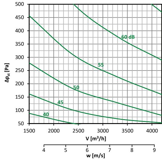
Diagramm nr. 37 – 500 × 250
