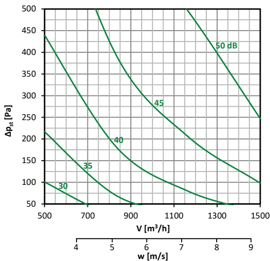
Diagramm nr. 51 – 300 × 150
