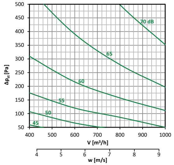
Diagramm nr. 2 – 200 × 150
