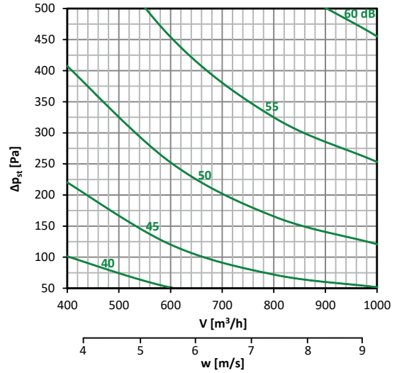
Diagramm nr. 27 – 300 × 100
