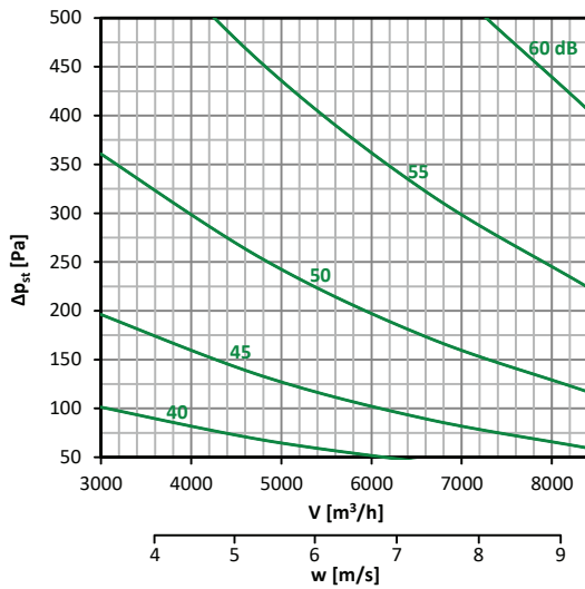
Diagramm nr. 63 – 500 × 500
