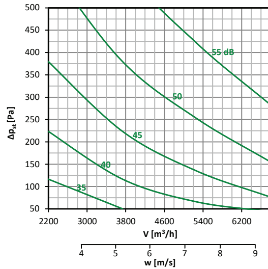
Diagramm nr. 62 – 500 × 400
