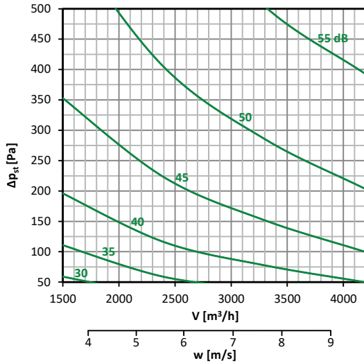
Diagramm nr. 57 – 400 × 300
