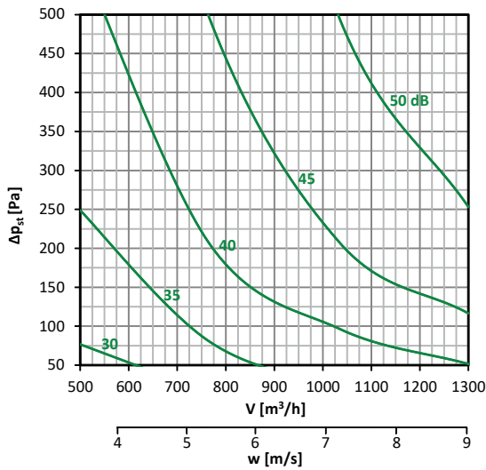
Diagramm nr. 49 – 200 × 200
