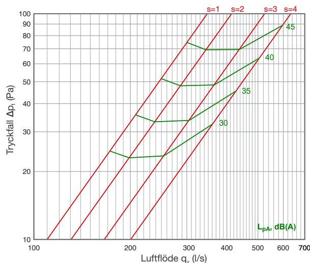
Frånluft: HU L=1500...1900
