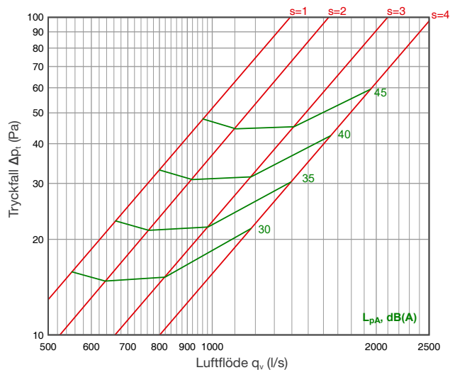
Frånluft: HU L=6000
