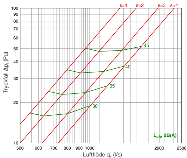
Frånluft: HU L=5000...5400
