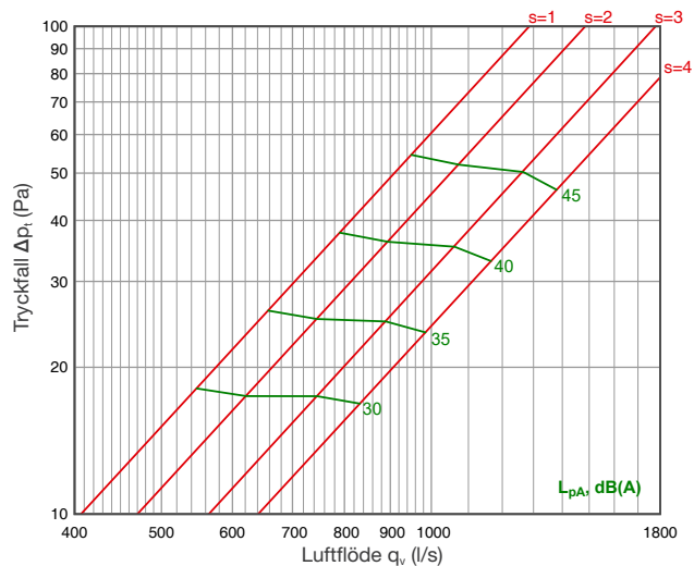
Frånluft: HU L=4000...4400
