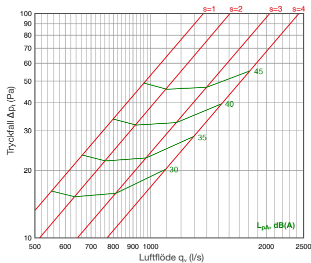
Frånluft: HU L=5500...5900
