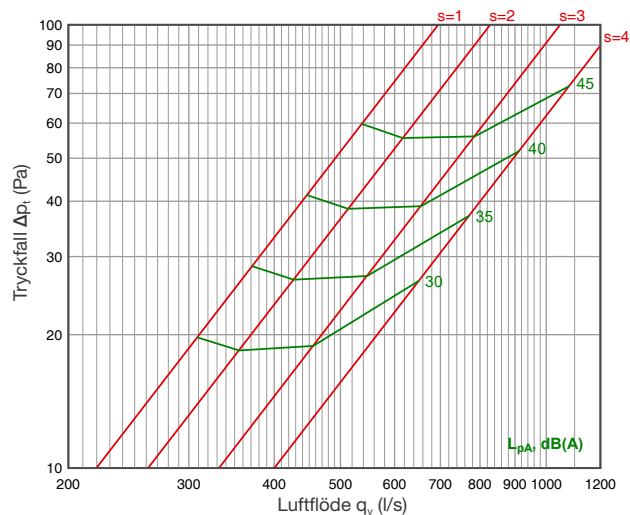
Frånluft: HU L=3000...3400
