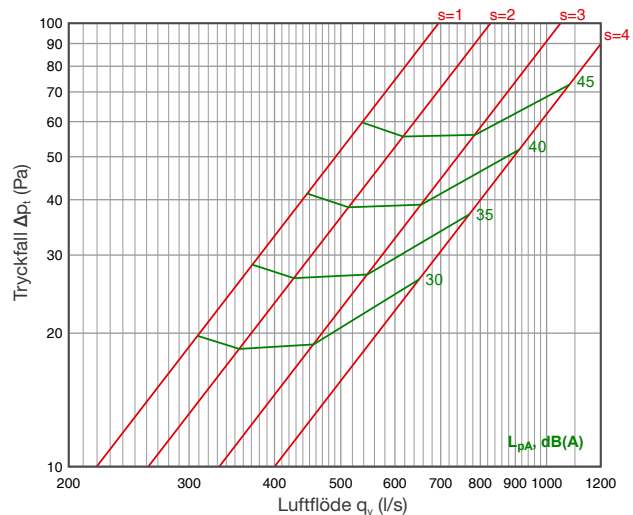
Frånluft: HU L=3500...3900
