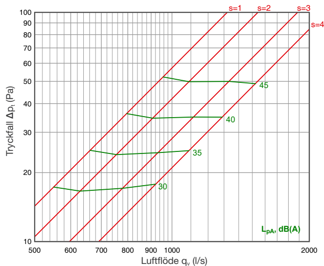
Frånluft: HU L=4500...4900
