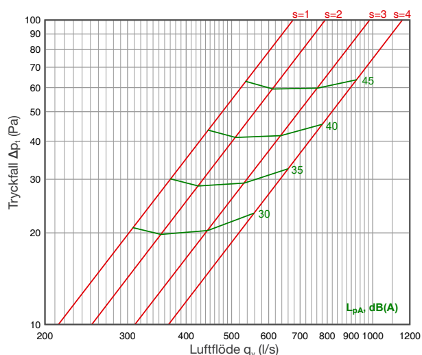
Frånluft: HU L=2500...2900
