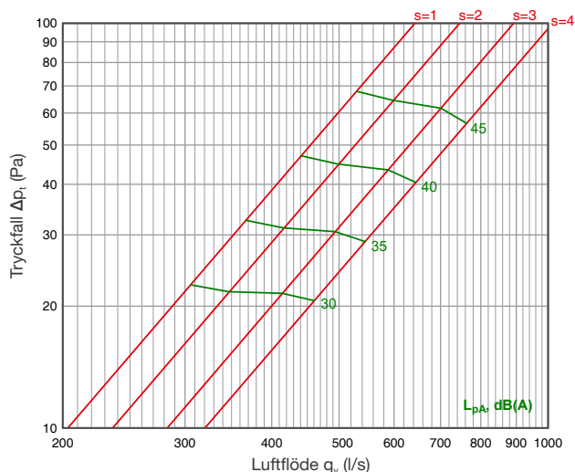
Frånluft: HU L=2000...2400
