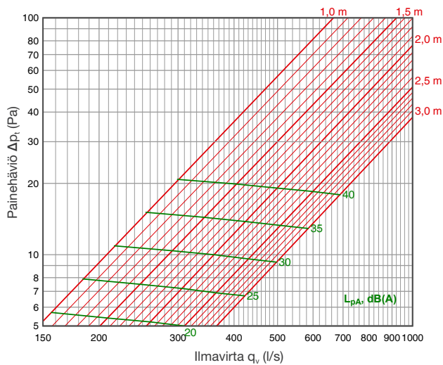
Tuloilma: SP×3+sivupaneelit
