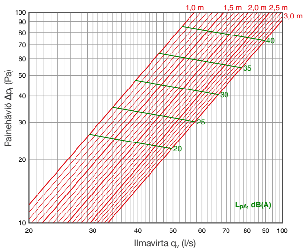
Tuloilma: "AirGrip"
