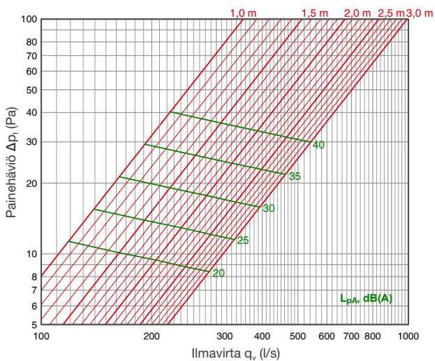
Tuloilma: SPx2
