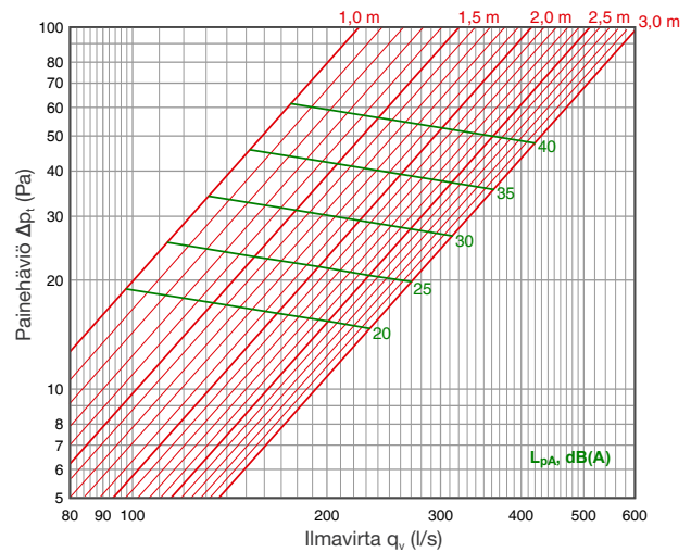
Tuloilma: SPx1
