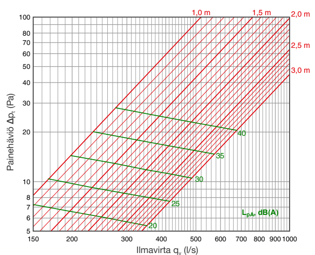
Tuloilma: SPx3
