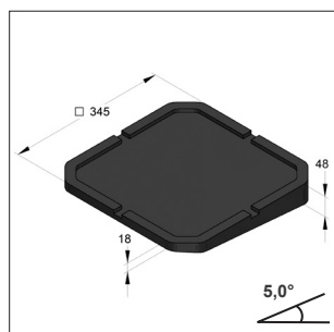
Rubber wedge 305 mm 5,0°
