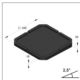
Rubber wedge 305 mm 2,5°
