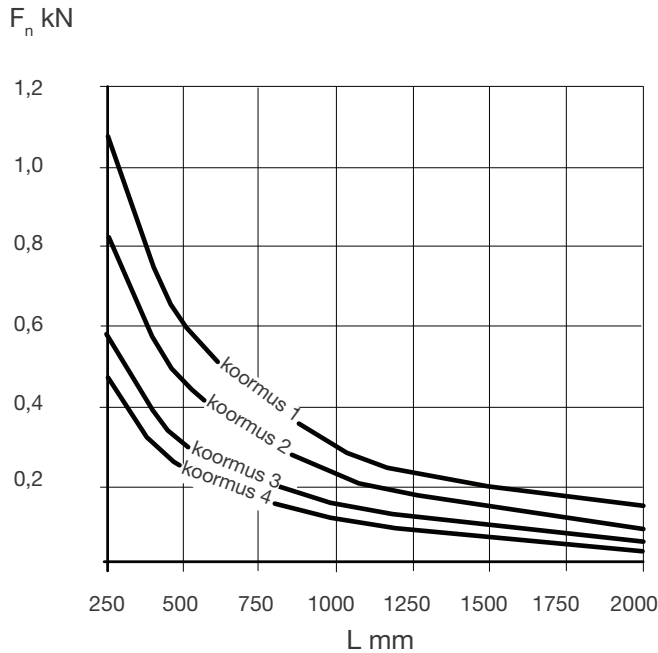
U-profiili 30x30x2 koormustabel
