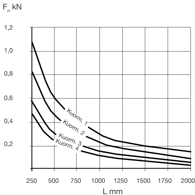
Kiskon U 30x30x2 kuormitustaulukko
