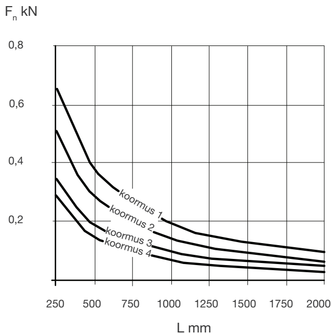
L-profiili 30x30x2 koormustabel
