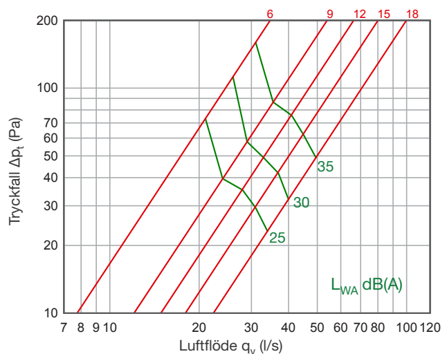
SFU 125
