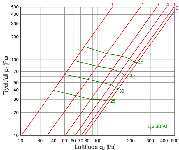
DEP 315 + SKDM 250/315
