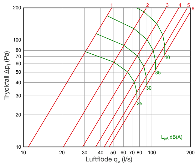
DEK 200 + SKDM 160/200
