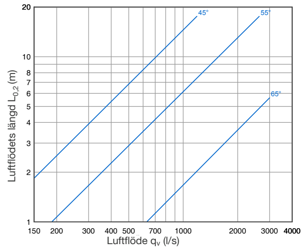
DPL 630 -15K
