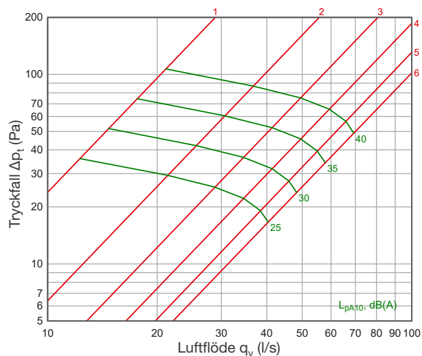
DEZ 125
