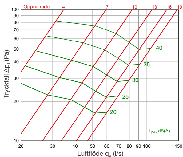
DSK 200
