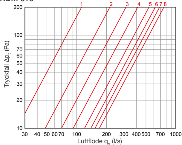
SKDM 315
