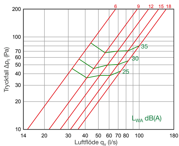
SFU 200
