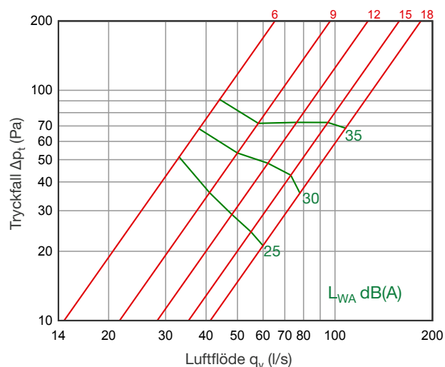
SFU 200
