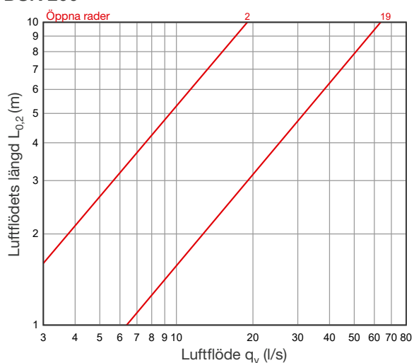
DSK 200
