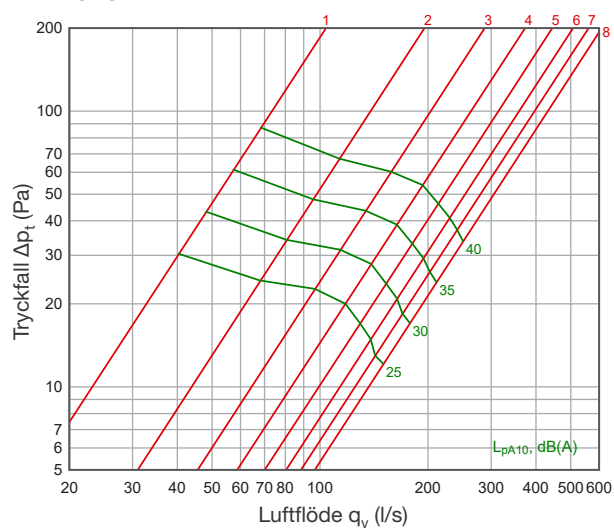
DEZ 315
