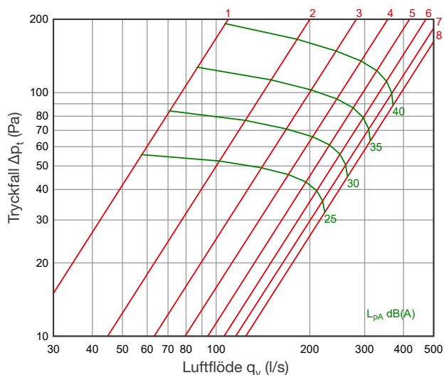
DEK 400 + SKDM 315/400
