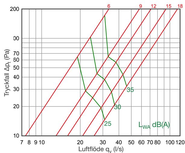
SFU 125
