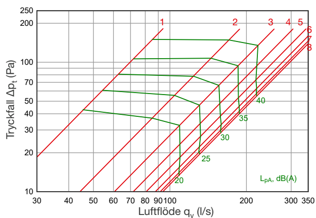
DEN 315
