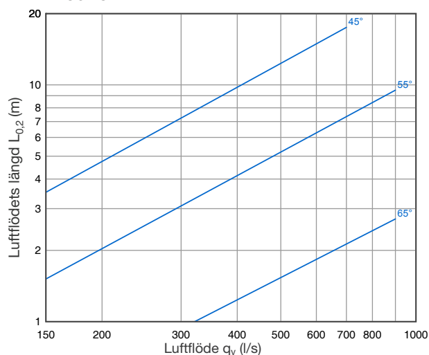
DPL 250 -5K
