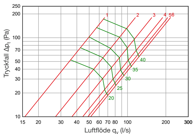
DEN 315
