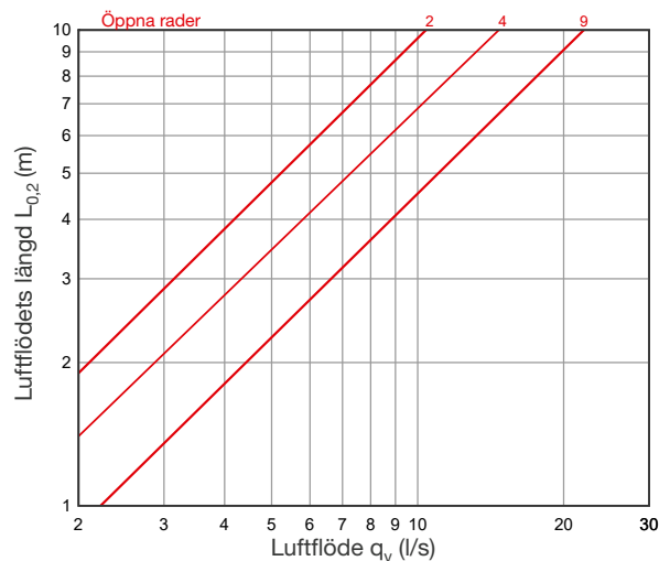
DSK-P2 100
