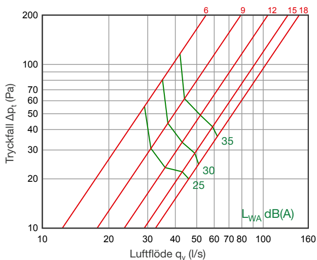
SFU 160
