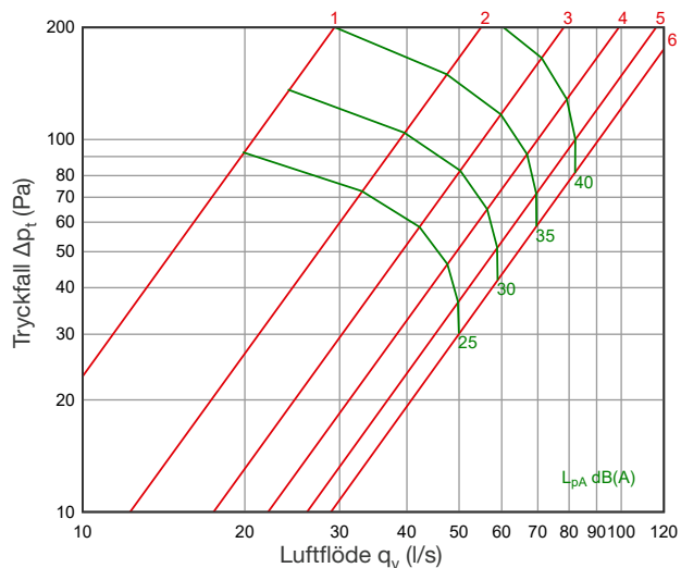
DEK 160 + SKDM 125/160
