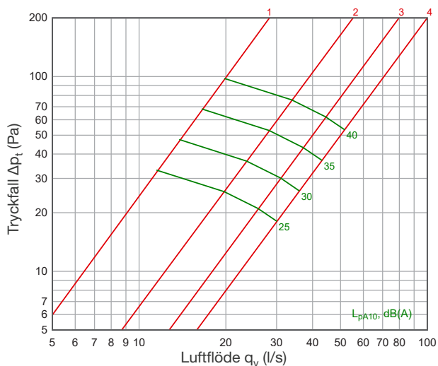
DEZ 100
