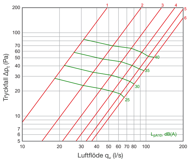
DEZ 160
