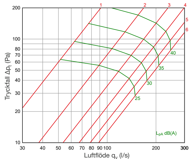
DEK 315 + SKDM 250/315
