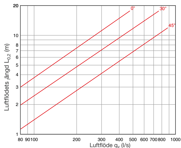
DPL 315 +5K
