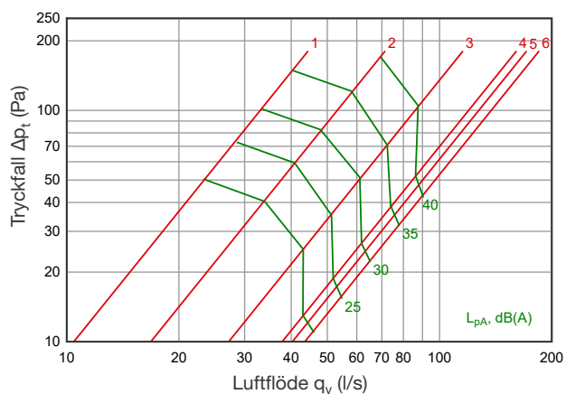
DEN 250
