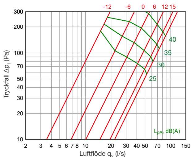
DSE 160
