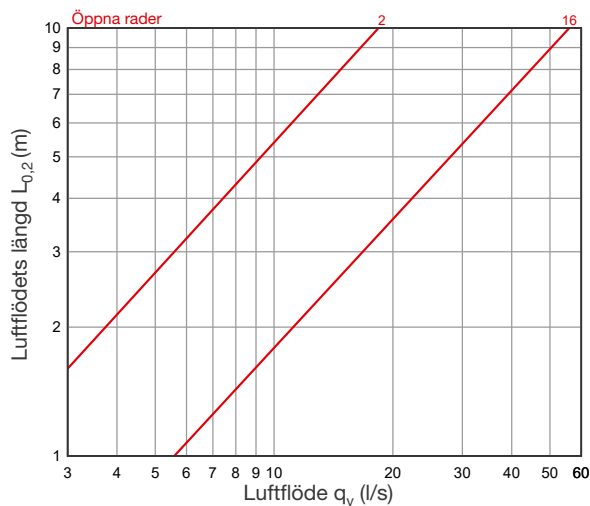
DSK 160
