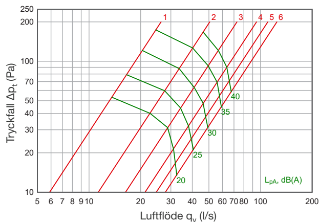
DEN 125
