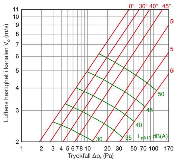
DPL 250 -5K
