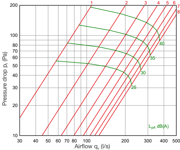
DEK 400 + SKDM 315/400
