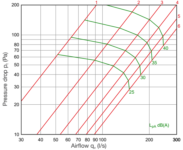
DEK 315 + SKDM 250/315
