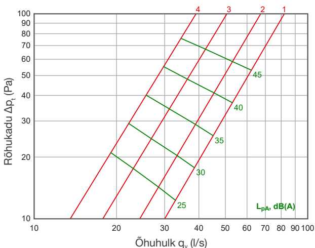
MRO 200×100
