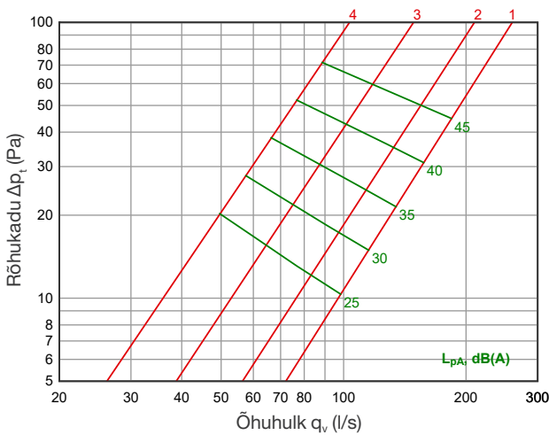
MRO 400×150
