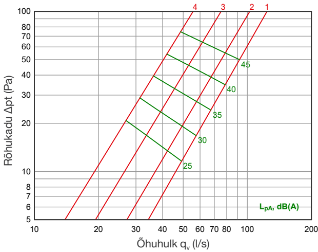
MRO 300×100
