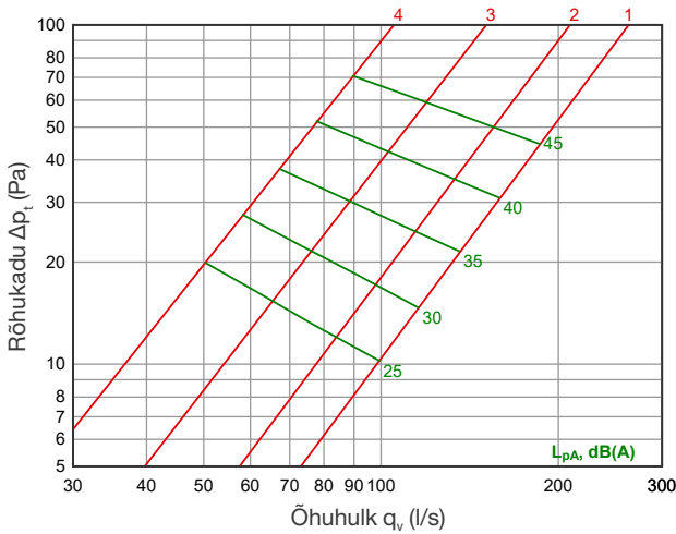
MRO 300×200
