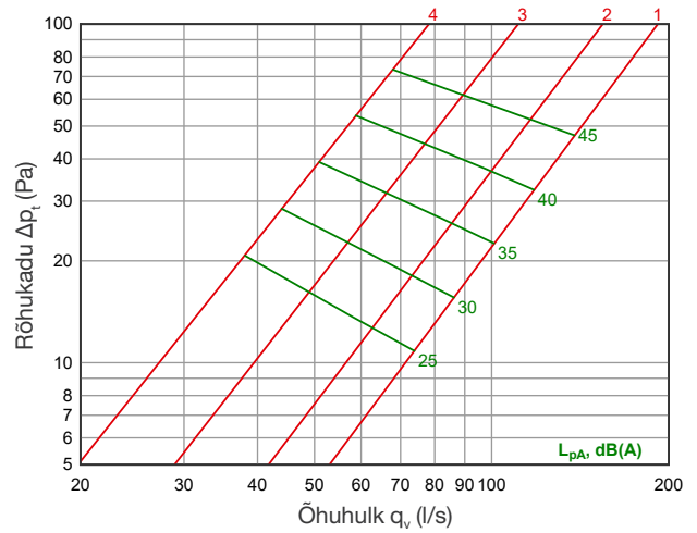
MRO 300×150
