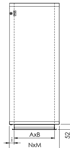
MKL-E20/E30/Z E20-europrofiiliga ühendus E30-europrofiiliga ühendus Z-profiiliga ühendus
