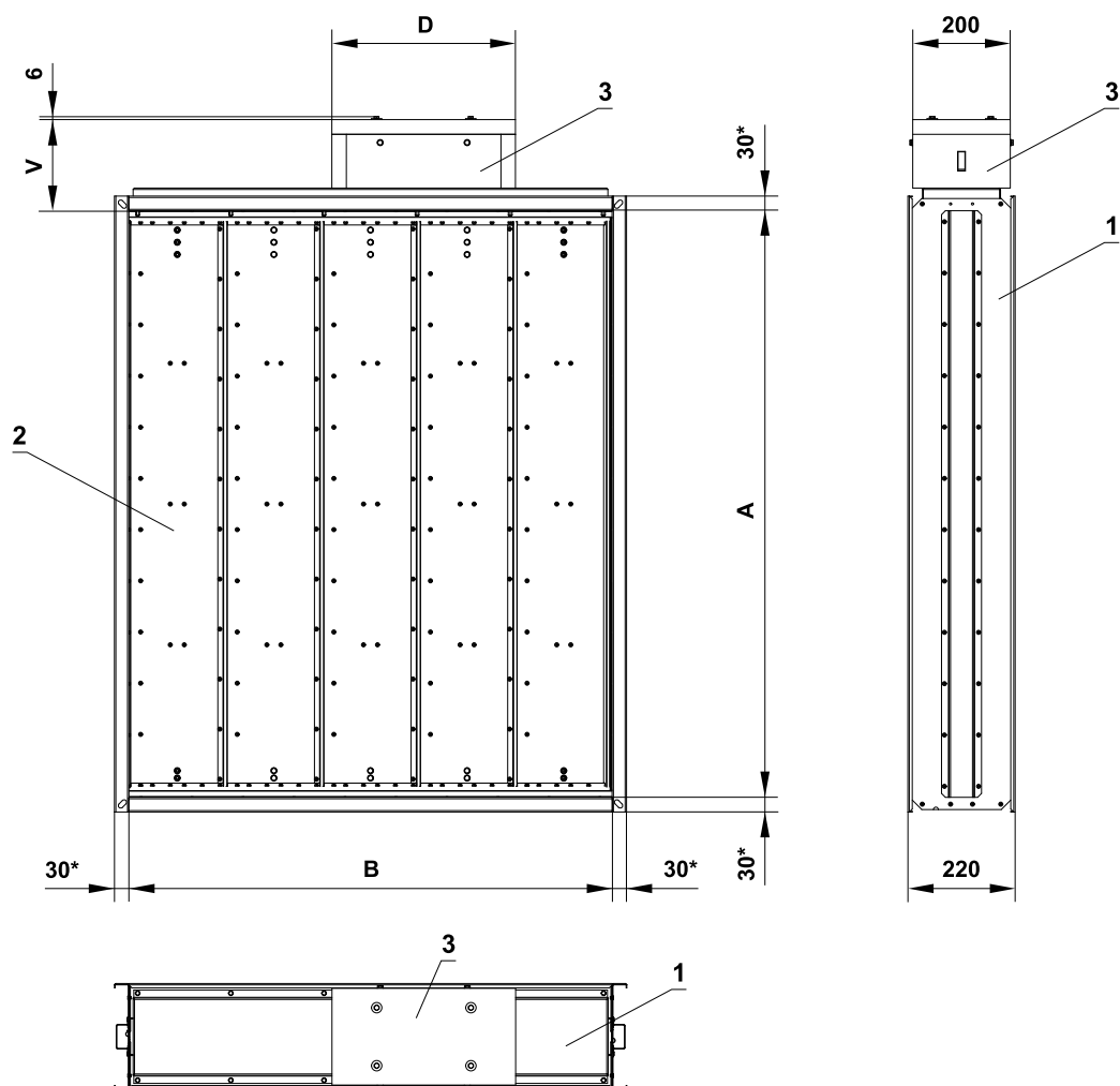
Fig. 10 Damper SEDS-L
