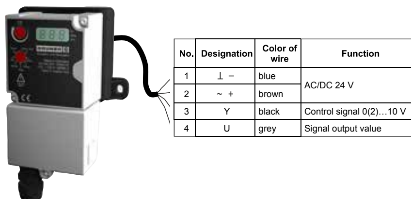
Fig. 21 Regulatory GUAC-...
